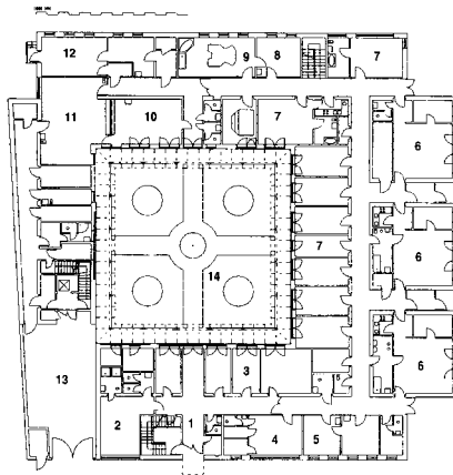
Půdorys přízemí
